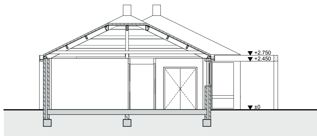
DOORSNEDE C
