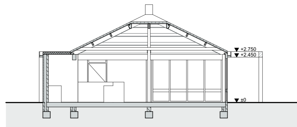
DOORSNEDE D
