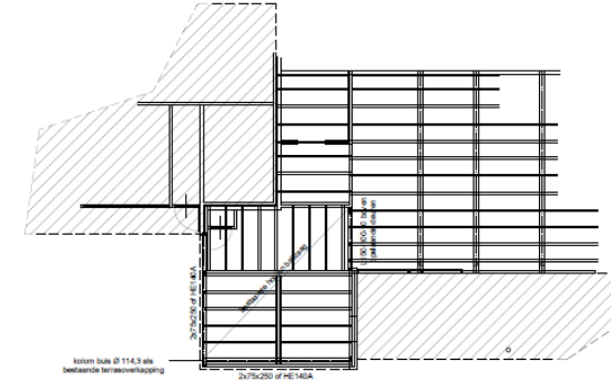
KAPPLAN
